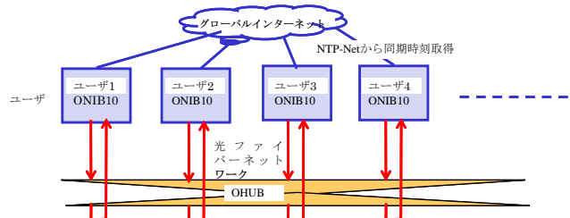
図2 本開発の光 LAN の構成
